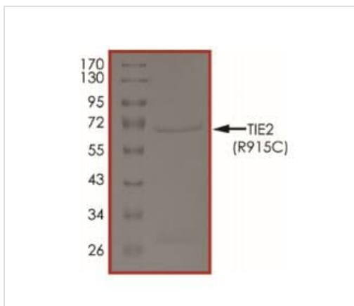
SDS-PAGE - (ab269048)
